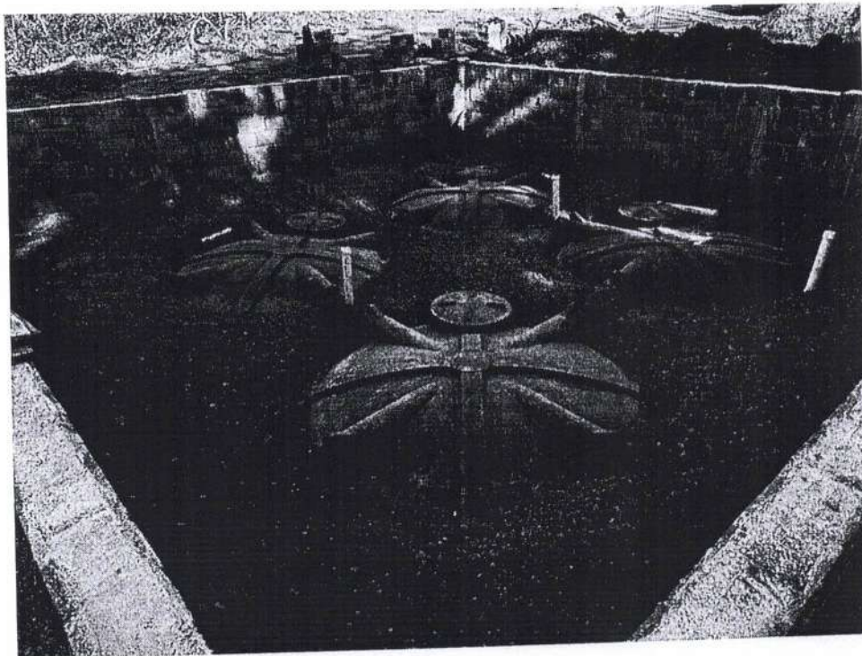
FOTO 02: REATORES ANAERÓBIOS.
