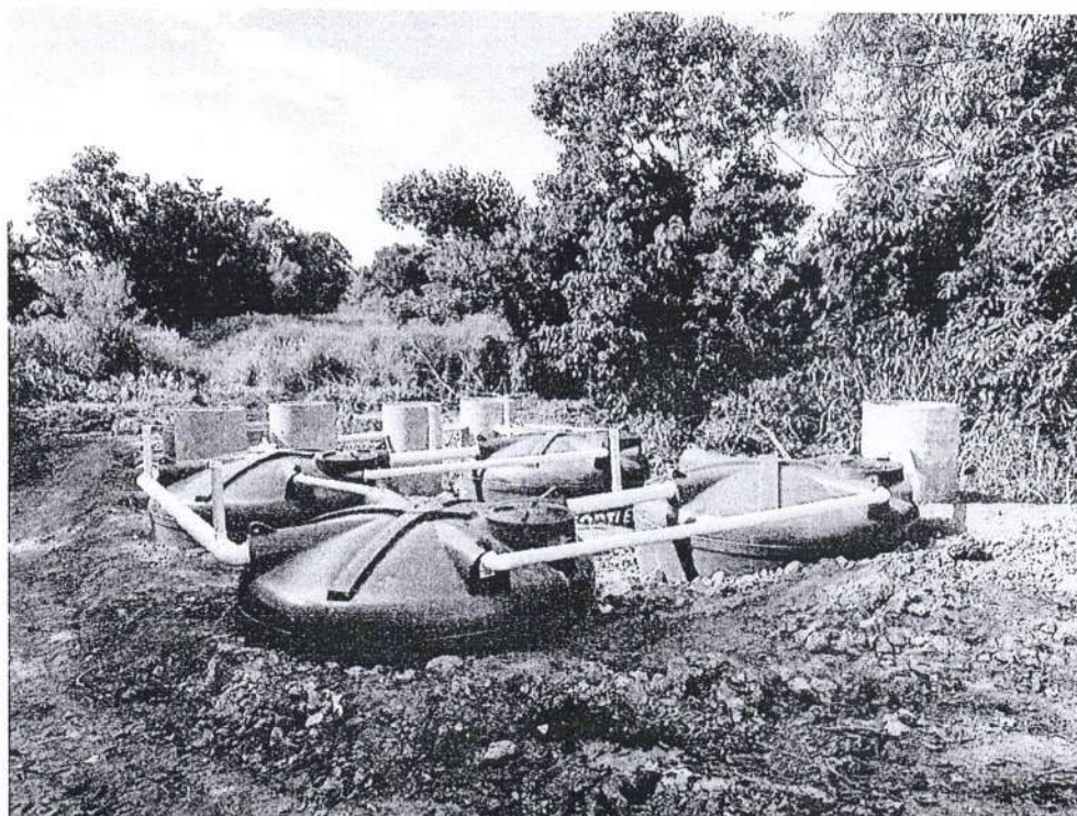
FOTO 03: TRATAMENTO PRELIMINAR, REATORES E FILTROS INSTALADOS.
